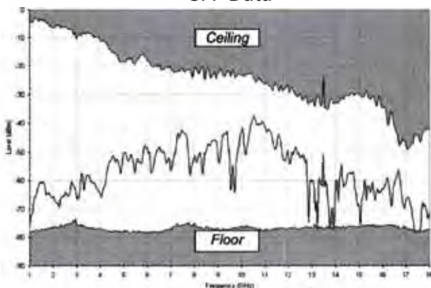
SFP Data
